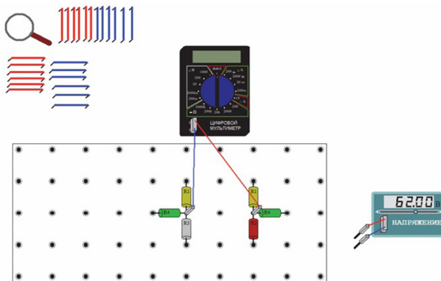
3-сурет. Модель «Алты дәнекерленген резистор және мультиметр»
